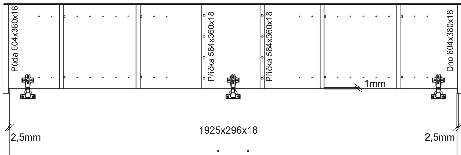
Boční pohled
