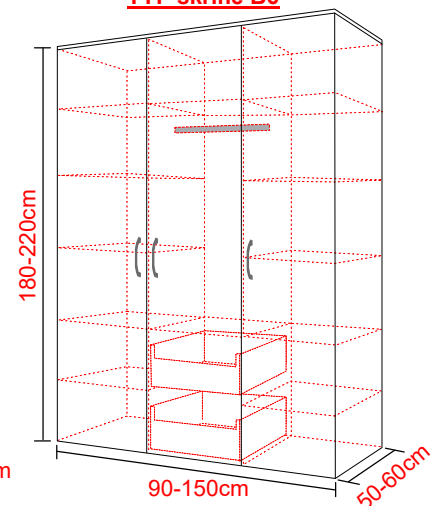
TYP skříně B6
