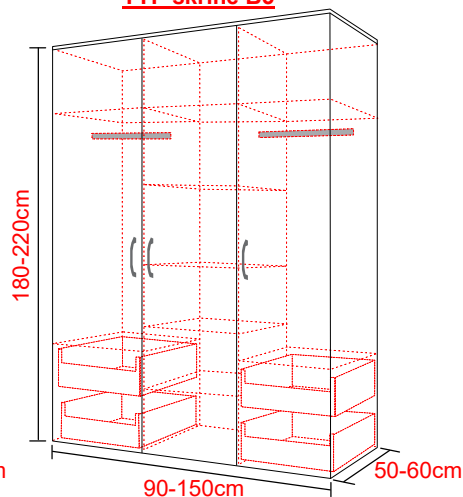
TYP skříně B5
