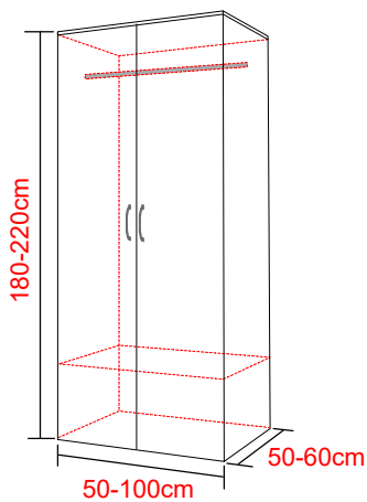
TYP skříně A1
