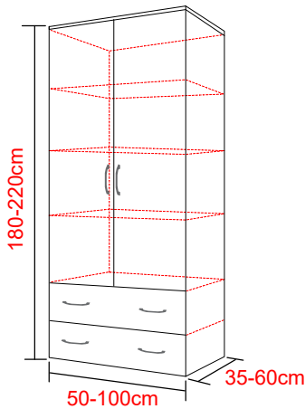
TYP skříně A6
