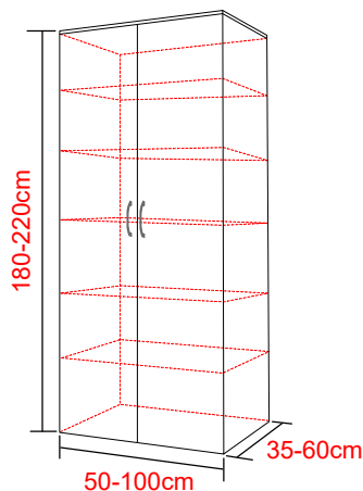
TYP skříně A4
