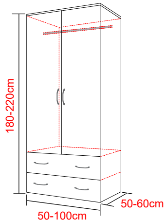
TYP skříně A5
