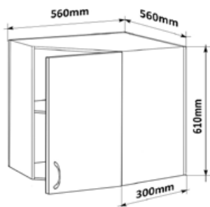
Horní rohová skříňka PL-P 56 LESK HNROH P 56x61x56
