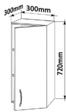
Skříňka horní PD 30 pravé LESK HORPL P 30x72x30
