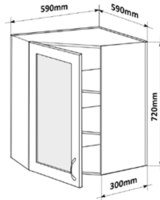
Horní rohová skříňka SK-L 59 LESK HVROH SKL L 59x72x59
