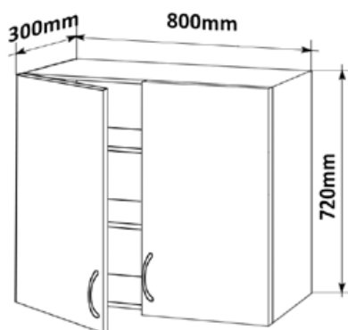
Skříňka horní PD 80 LESK HORPL 80x72x30
