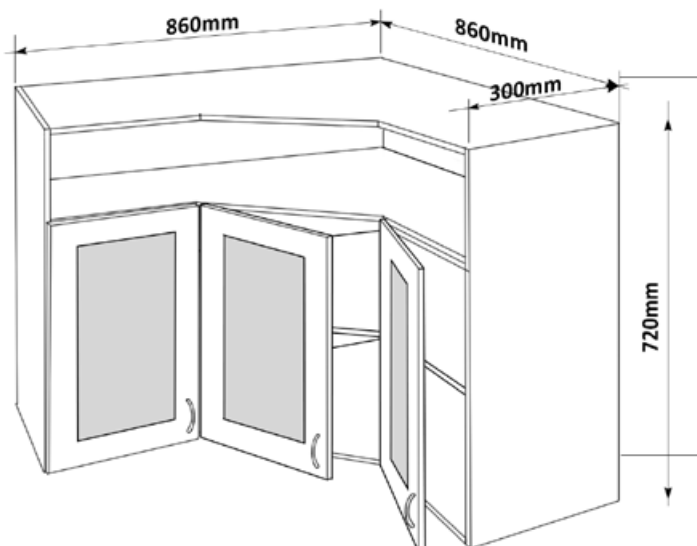
Rohová skříňka horní levá LESK ROH SKL L 86x72x86
