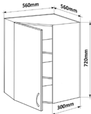
Horní rohová skříňka PL-L 56 LESK HVROH L 56x72x56
