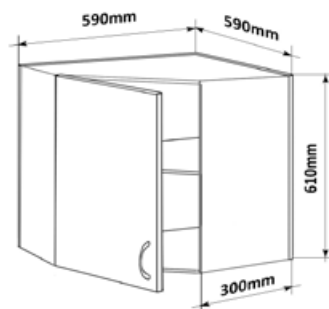
Horní rohová skříňka PL-L 59 LESK HNROH L 59x61x59
