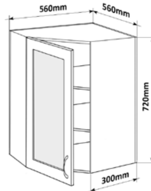
Horní rohová skříňka SK-L 56 LESK HVROH SKL L 56x72x56
