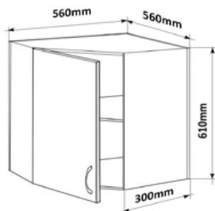
Horní rohová skříňka PL-L 56 LESK HNROH L 56x61x56
