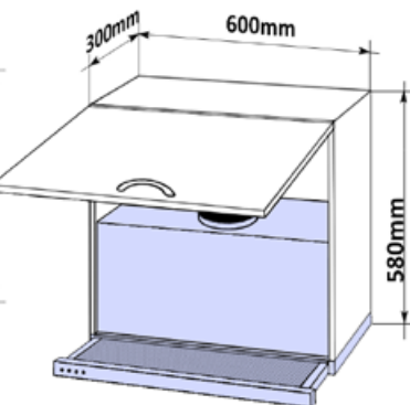
LESK VYS DIG 60x58x30
