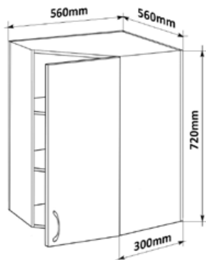
Horní rohová skříňka PL-P 56 LESK HVROH P 56x72x56
