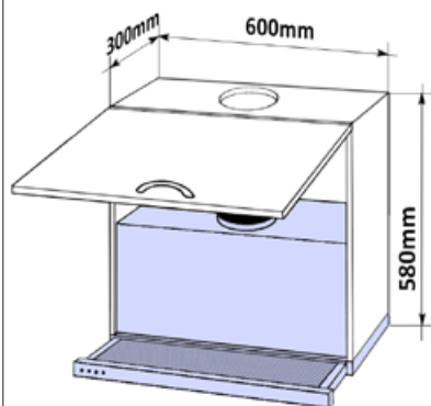
LESK VYS DIG OT 60x58x30
