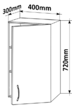
Skříňka horní PD 40 pravé LESK HORPL P 40x72x30
