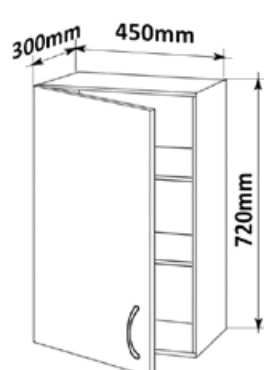
Skříňka horní PD 45 levé LESK HORPL L 45x72x30
