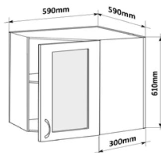
Horní rohová skříňka SK-P 59 LESK HNROH SKL P 59x61x59
