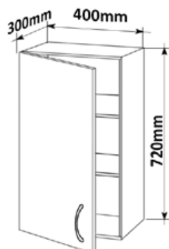
Skříňka horní PD 40 levé LESK HORPL L 40x72x30
