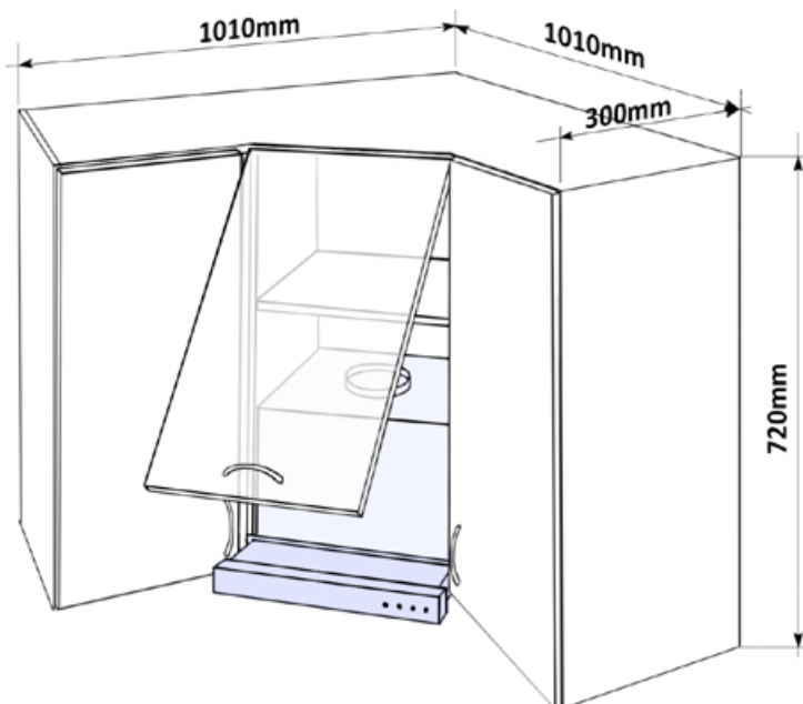
LESK ROH VYS DIG 101x72x101
