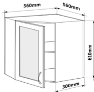
Horní rohová skříňka SK-L 56 LESK HNROH SKL L 56x61x56
