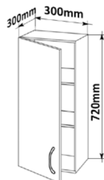
Skříňka horní PD 30 levé LESK HORPL L 30x72x30
