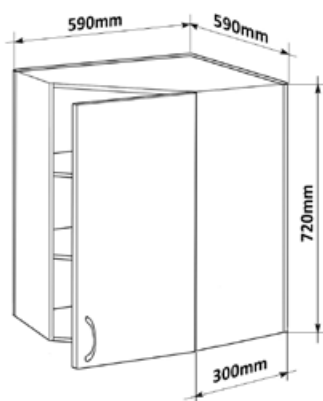
Horní rohová skříňka PL-P 59 LESK HVROH P 59x72x59
