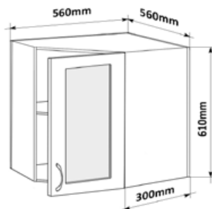
Horní rohová skříňka SK-P 56 LESK HNROH SKL P 56x61x56
