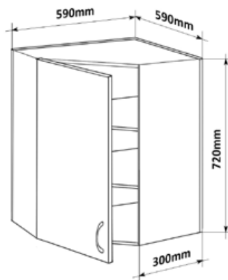
Horní rohová skříňka PL-L 59 LESK HVROH L 59x72x59
