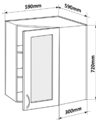
Horní rohová skříňka SK-P 59 LESK HVROH SKL P 59x72x59
