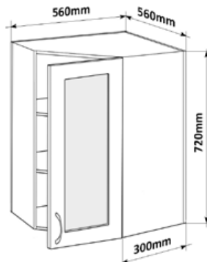
Horní rohová skříňka SK-P 56 LESK HVROH SKL P 56x72x56
