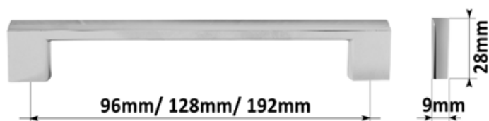
Úchytka chrom UV 3001 019 - 021
