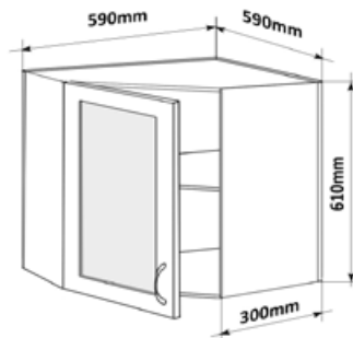
Horní rohová skříňka SK-L 59 LESK HNROH SKL L 59x61x59
