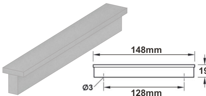
Úchytka plast 128 - lak
