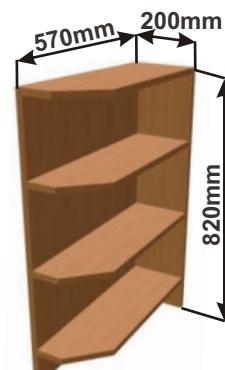
Police rohová pravá LAM ROPO P 20x82x57
