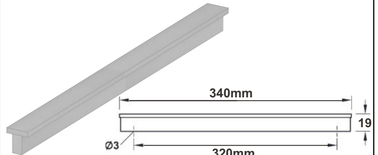
Úchytka plast 320 - lak
