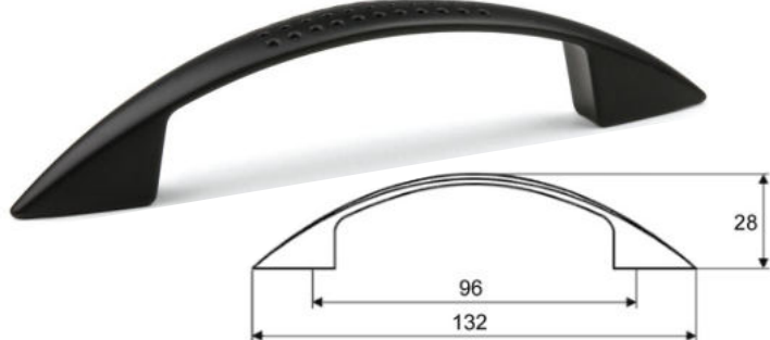
Úchytka Ruona 96 - černá
