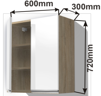
Skříňka horní PD 60 HORPL 60x72x30
