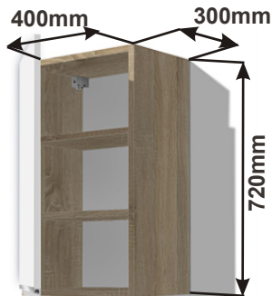
Skříňka horní PD 40 levé HORPL L 40x72x30
