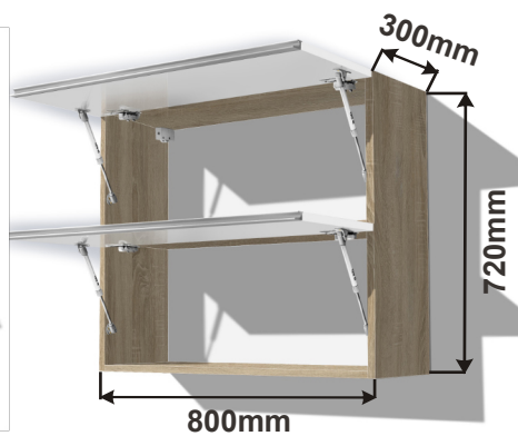
Skříňka horní HORPL 80 80x72x30
