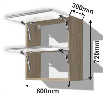
Skříňka horní HORPL 60 HK-XS 60x72x30
