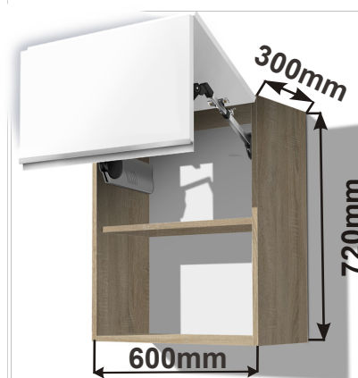
Skřínka horní lomené HF 60 HORPL 60x72x30 BLUM
