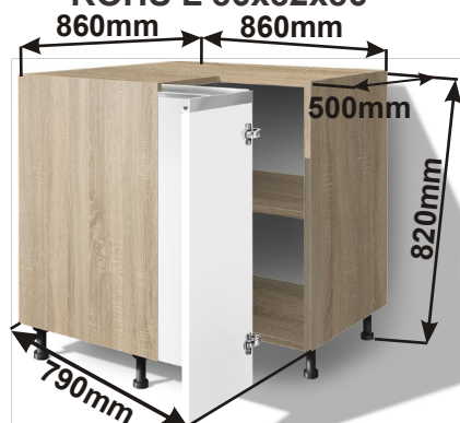
Skříňka roh.lomené dv. levé ROHS L 86x82x86
