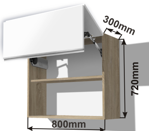
Skřínka horní lomené HF 80 HORPL 80x72x30 BLUM
