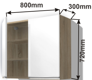
Skříňka horní PD 80 HORPL 80x72x30
