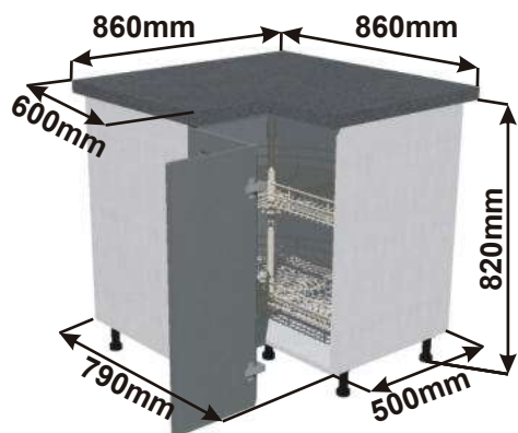
Spodní roh ODP levá RET ROH ODP 690/3-4 L 86x82x86
