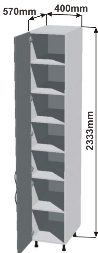
Skříňka 40 levá RET VYS L 40x233,3x57
