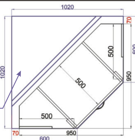
Police rohová pravá LAM ROPO P 20x82x57
