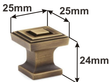
Úchytka SERENA knopek - staroměď matná
