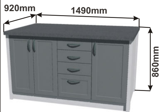
Pohled zepředu
