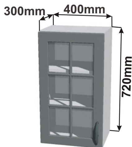
Skříňka prosklená 40 L RET HOR SKL L 40x72x30
