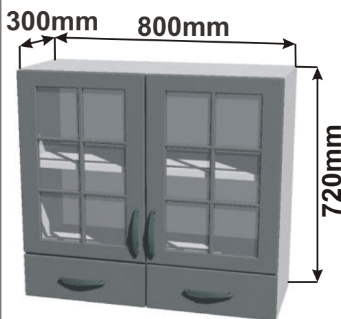
Skříňka prosklená 80 RET HOR SKL ZAS 80x72x30
