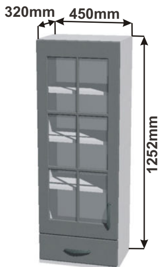
Skříňka horní kredenc 45 L RET HORKR L 45x125,2x32 1Z
