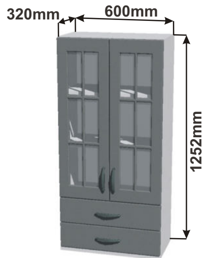
Skříňka horní kredenc 60 RET HORKR 60x125,2x32 2Z
