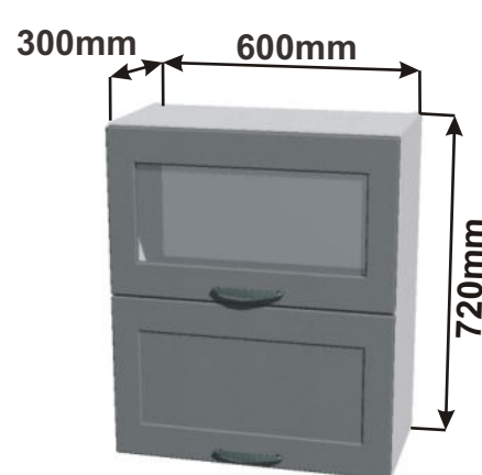
Skříňka horní HP60 RET HV SKL 60x72x30
