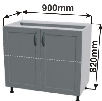
Skříňka 90 RET SPO 90x82x50
