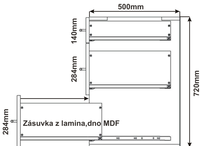
Boční pohled
