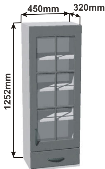
Skříňka horní kredenc 45 P RET HORKR P 45x125,2x32 1Z
