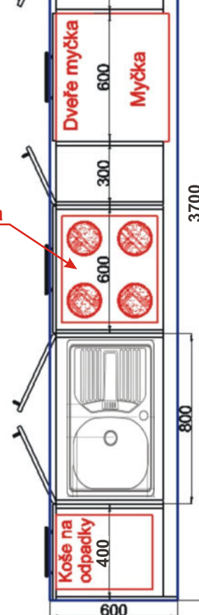
Varná deska
