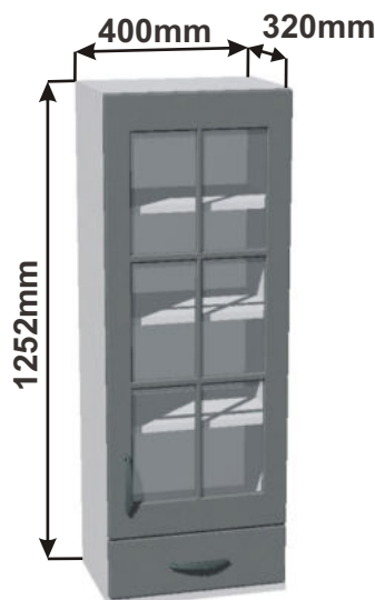
Skříňka horní kredenc 45 P RET HORKR P 40x125,2x32 1Z
