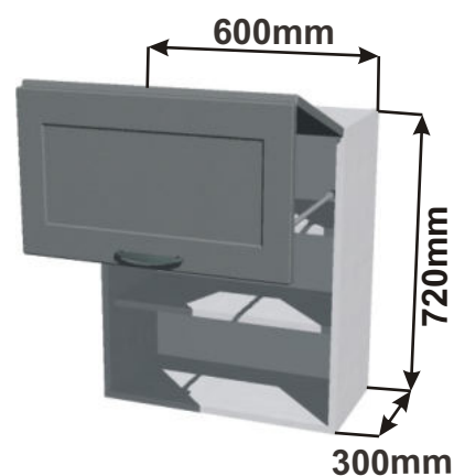
Skřínka horní lomené HF 60 RET HORPL 60x72x30
