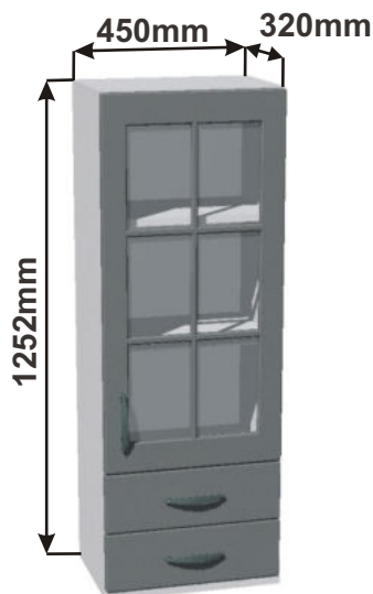
Skříňka horní kredenc 45 P RET HORKR P 45x125,2x32 2Z
