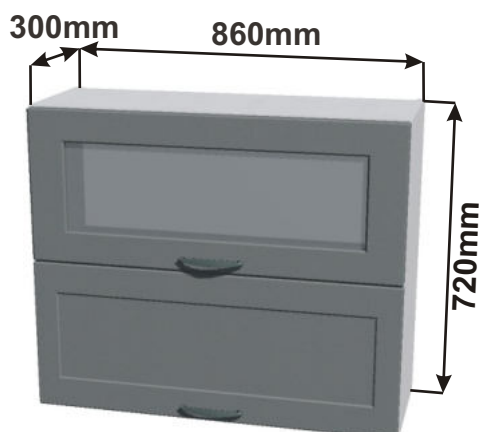
Skříňka horní HP86 RET HV SKL 86x72x30
