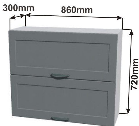
Skříňka horní HPLN 86 RET HV PLN 86x72x30
