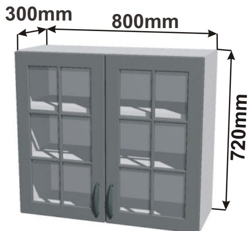
Skříňka prosklená 80 RET HOR SKL 80x72x30
