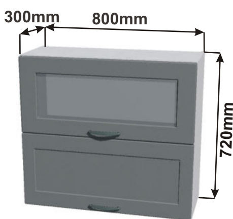
Skříňka horní HP80 RET HV SKL 80x72x30
