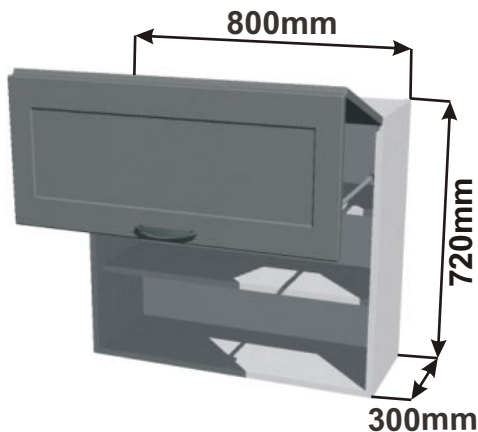
Skřínka horní lomené HF 80 RET HORPL 80x72x30
