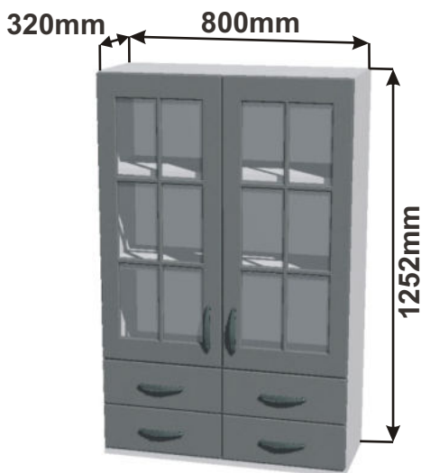
Skříňka horní kredenc 80 RET HORKR 80x125,2x32 4Z
