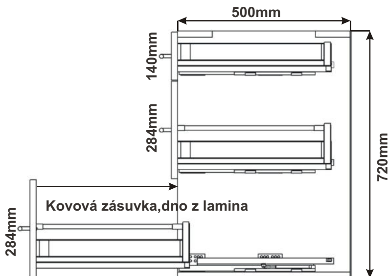
Boční pohled
