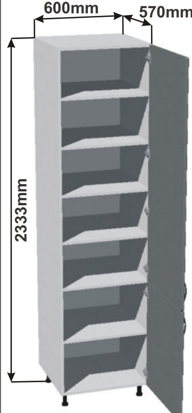
Skříňka 60 pravá RET VYS P 60x233,3x57
