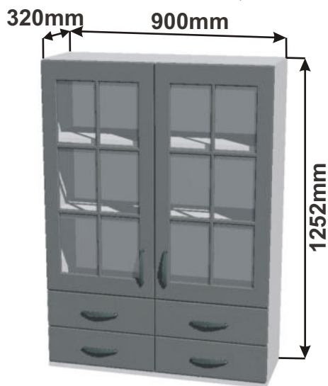
Skříňka horní kredenc 90 RET HORKR 90x125,2x32 4Z
