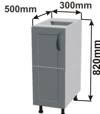
Skříňka 30 levá RET SPO L 30x82x50
