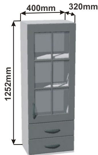
Skříňka horní kredenc 45 P RET HORKR P 40x125,2x32 2Z
