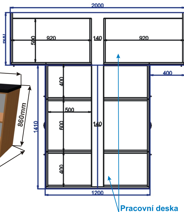
Půdorys
